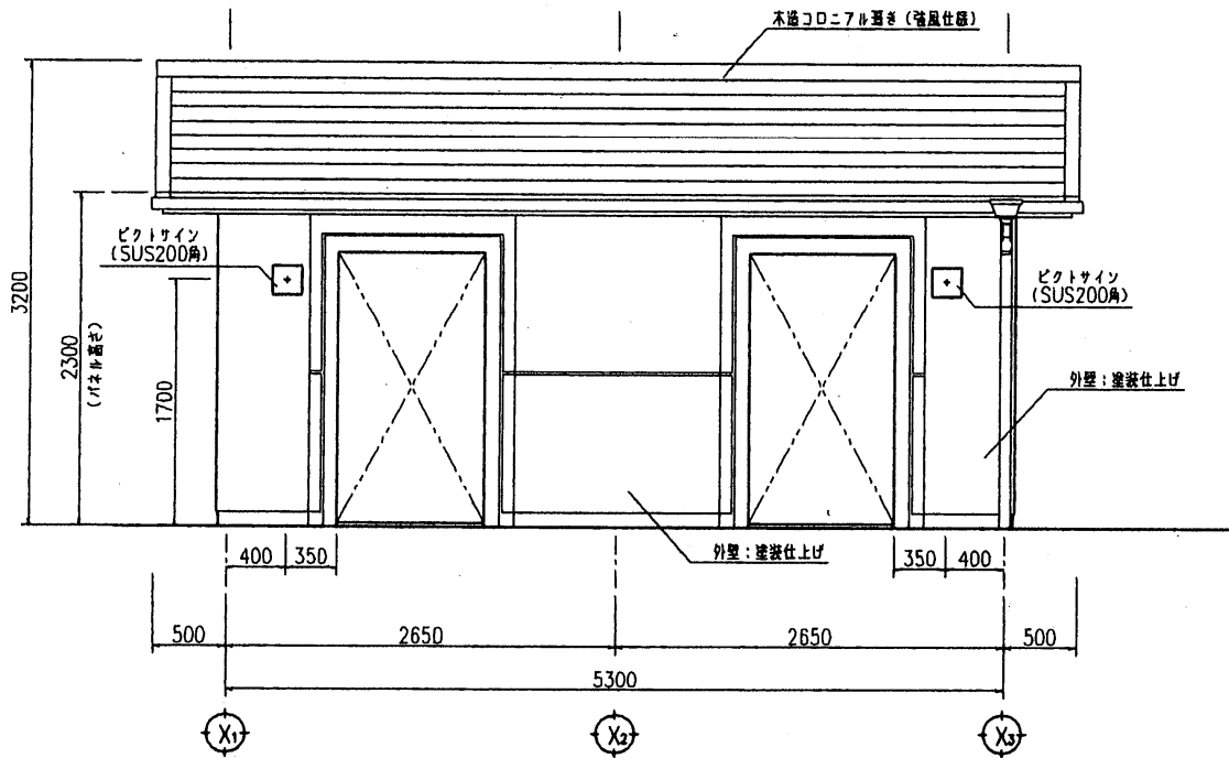
正面立面図 S: 1/50
