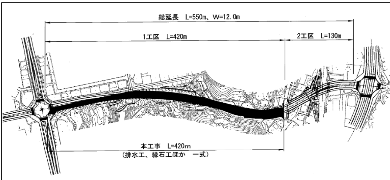
陣内・白野線 計画図
