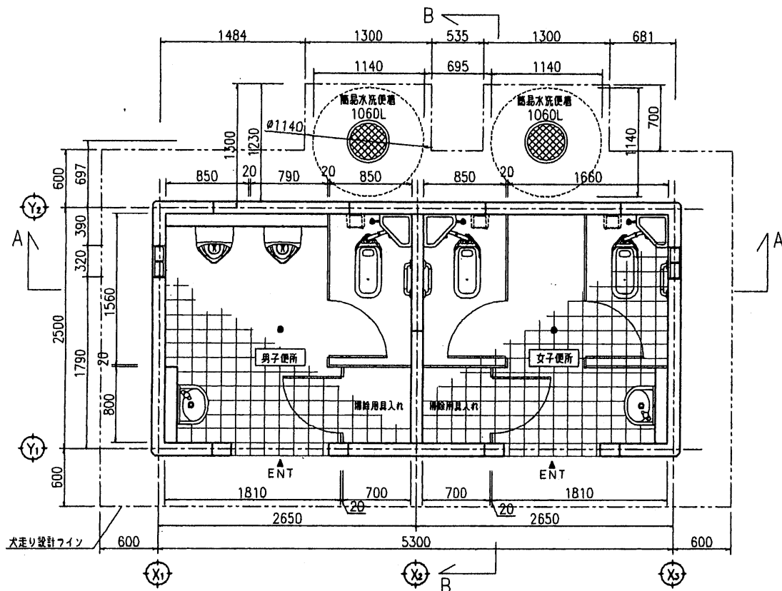
平面図 S: 1/50
