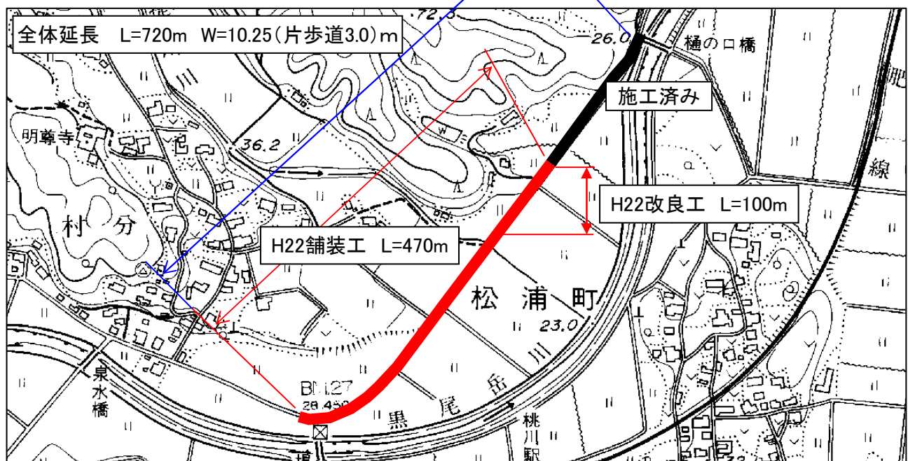
市道提川・川西線 計画図
