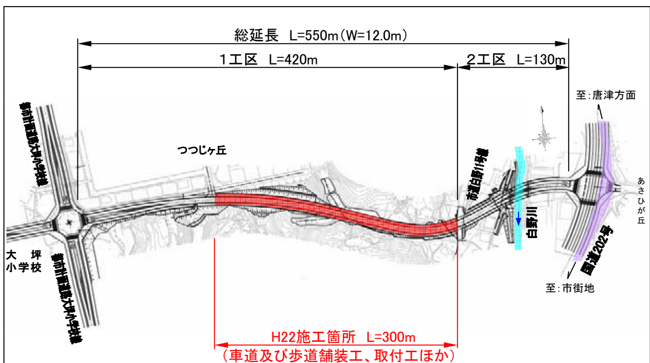
陣内・白野線 計画図
