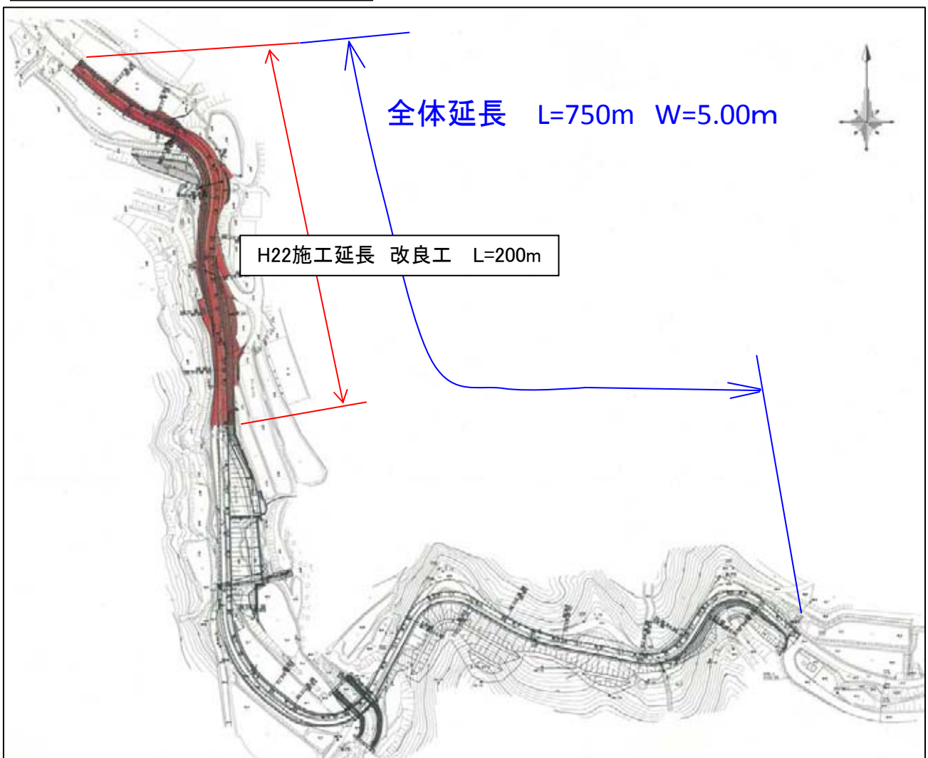
市道竹の古場・世知原線 計画図
