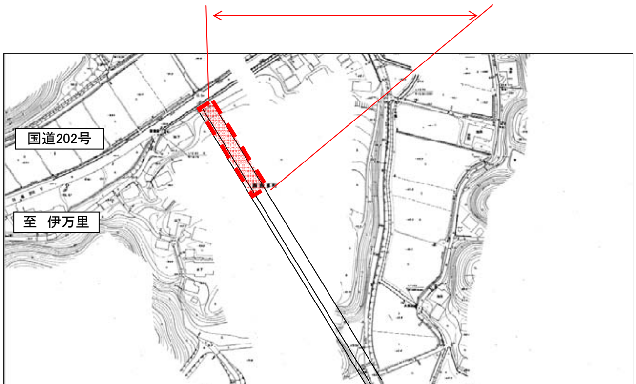
市道府招・藤川内線 計画図
