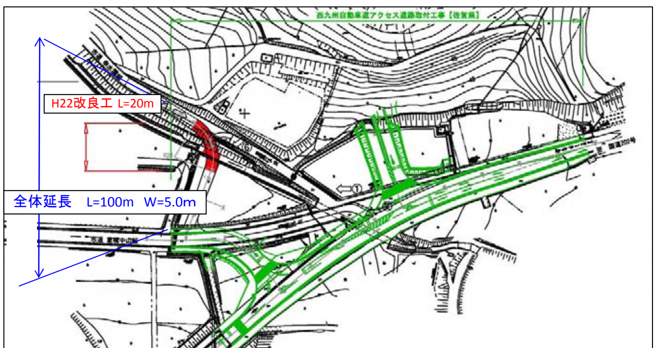
市道幸水園線 計画図
