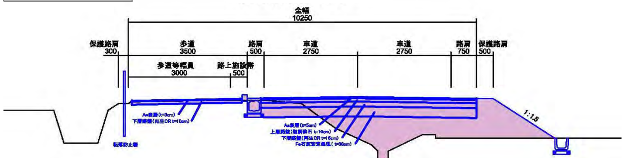
標準断面図
