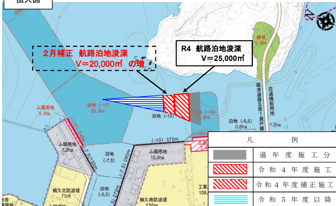
拡大図
