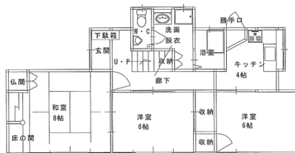
1 階
