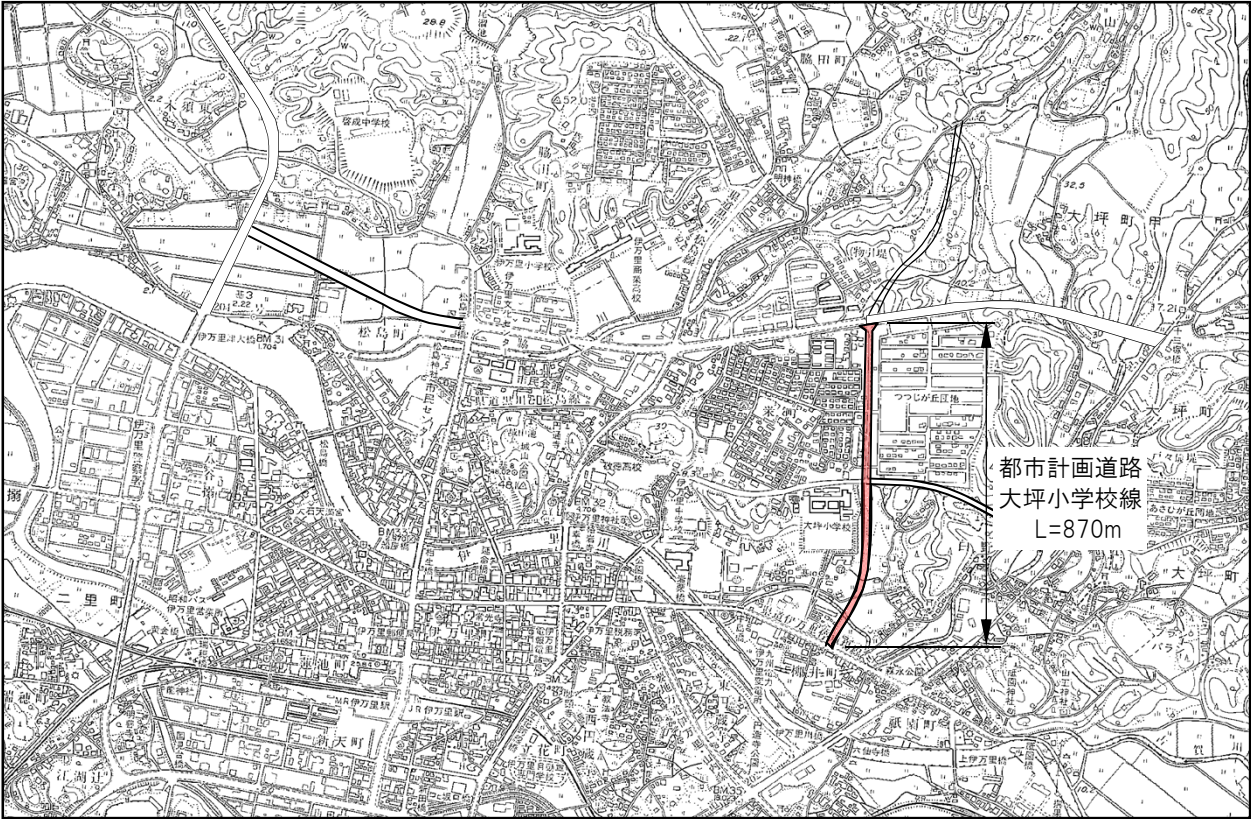
大坪小学校線 計画図
