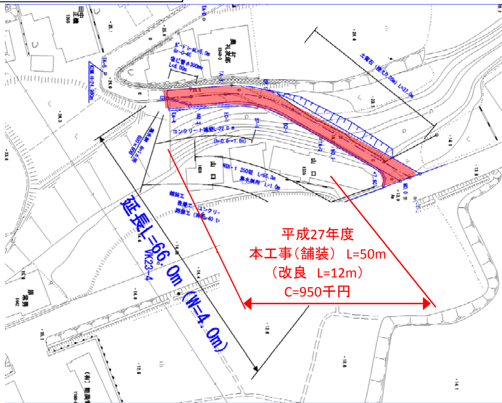
六仙寺5号線 計画図
