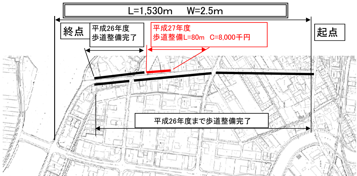
八谷搦海岸通り線 計画図
