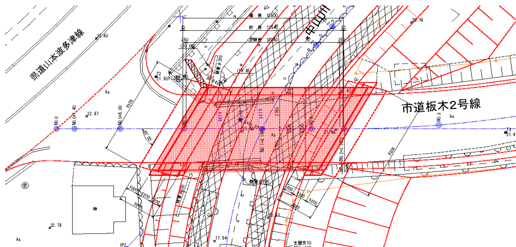
小の原橋 計画図
